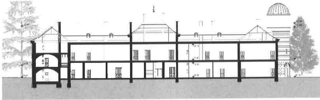
A-A metszet
